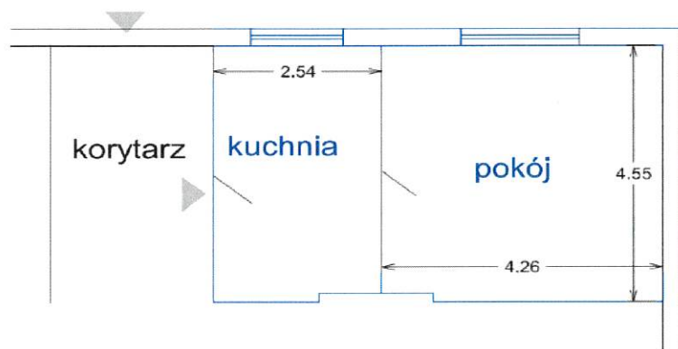
Rysunek: Rzut lokalu mieszkalnego
